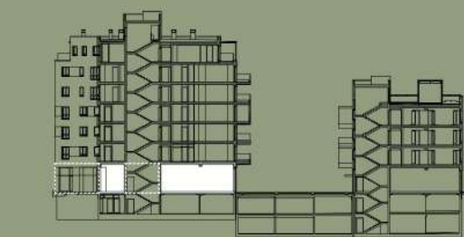
presjek 1:1000
