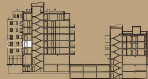
presjek 1:1000
