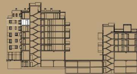
presjek 1:1000
