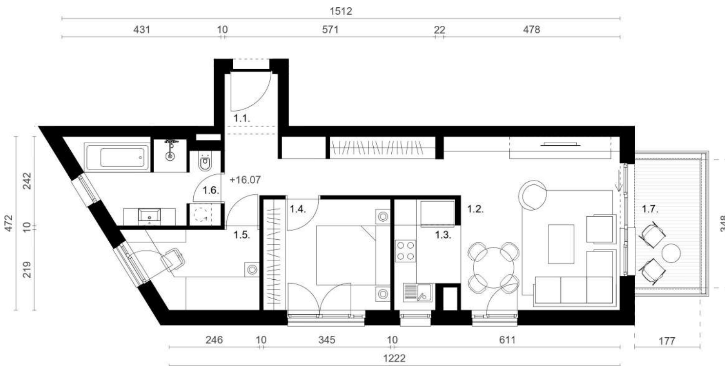
tlocrt 1:1000
